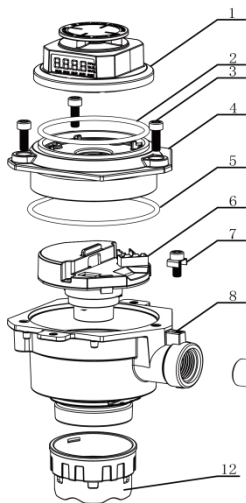
图 2-4 GTYQ-SST626SMG 组成结构示意图
