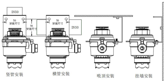
图 4-1 安装示意图
