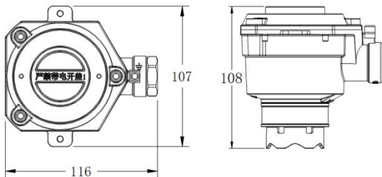
图 2-1 GTYQ-SST626LED 外形尺寸示意图（单位：mm）
